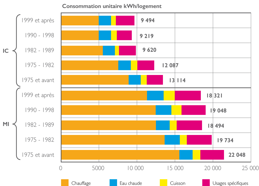
EVOLUTION DES CONSOMMATIONS ÉNERGÉTIQUES DES IMMEUBLES COLLECTIFS (IC) ET DES MAISONS INDIVIDUELLES (MI)
