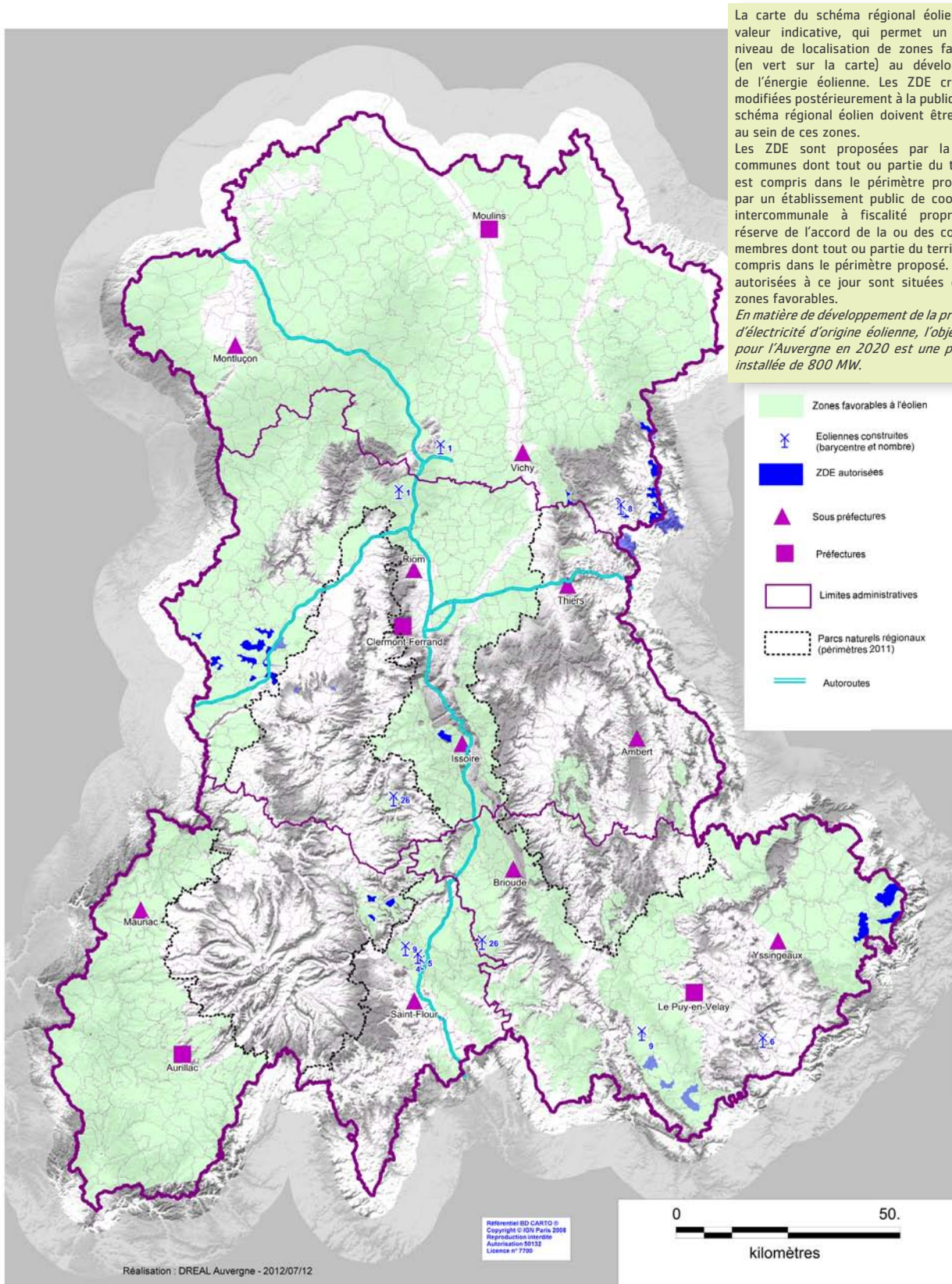
Figure n° 18 : Schéma régional éolien Auvergne : Proposition de zones favorables au développement de l'énergie éolienne en Auvergne
